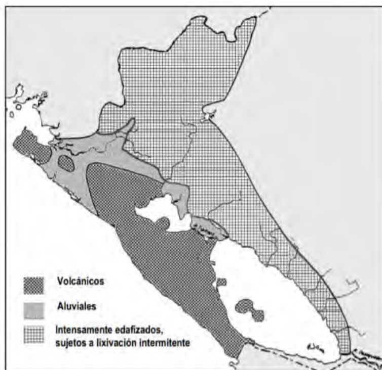
Figura 3. 10. Tipos de suelos del Sector norte de la Gran Nicoya. Modificado de Roser Solà (1986: 21).
