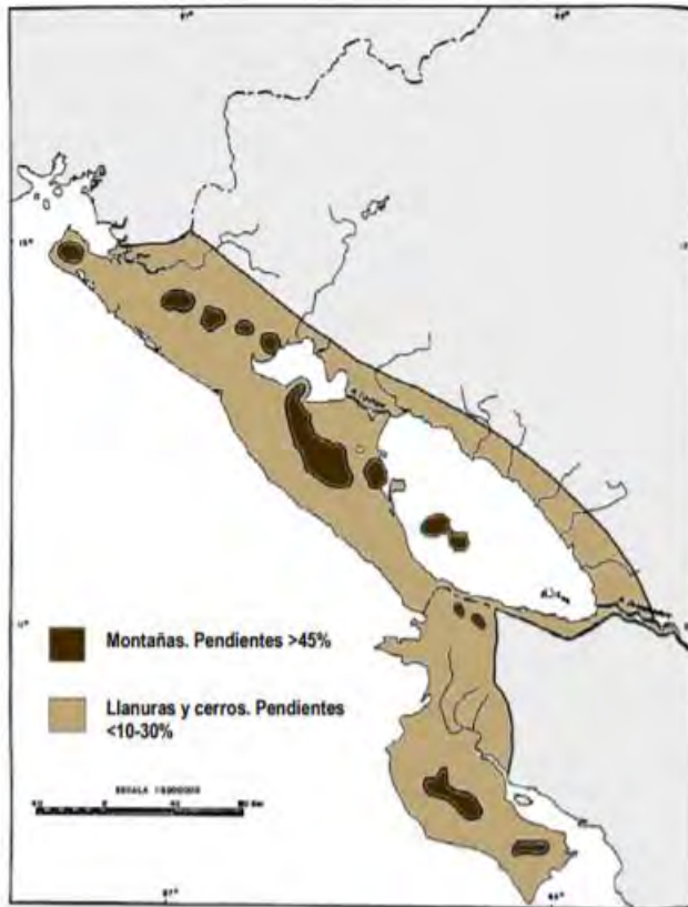
Figura 3. 7. Orografía de la Gran Nicoya. Modificado de Elisabeth Fonseca (1997: 27) y Roser Solà (1986: 15).
