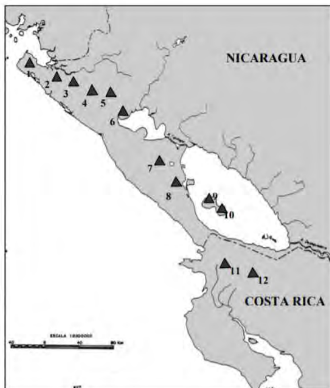
Figura 3. 8. Vulcanismo en la Gran Nicoya. 1. Cosigüina, 2. San Cristóbal, 3. Telica, 4. Las Pilas, 5. Hoyo, 6. Momotombo, 7. Masaya, 8. Mombacho, 9. Concepción, 10. Maderas, 11. Orosí, 12. Rincón de la Vieja. Modificado de Roser Solà (1986: 15).
