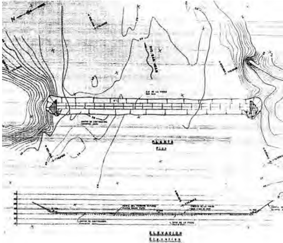
Figura 4- Planta y Elevación de la presa en el Río San Juan
