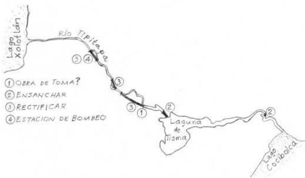
Figura 5 – Esquema de la conexión entre el lago Cocibolca y el lago Xolotlán
