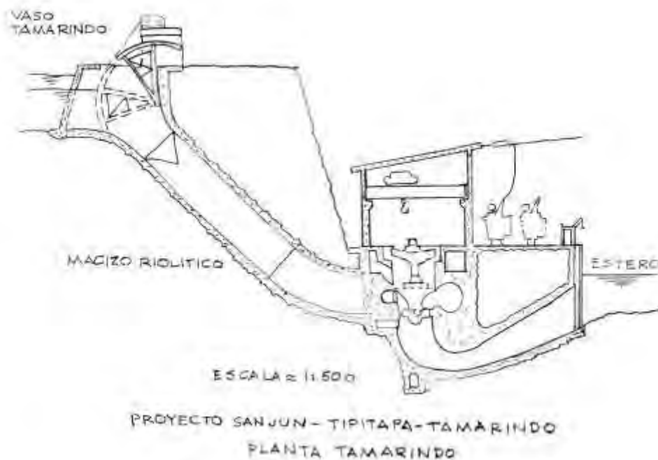
Figura 10 – Sección de la planta hidroeléctrica de 115 MW El Tamarindo
